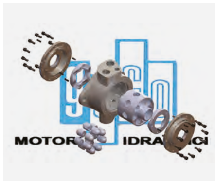
▲ Esploso motori SF.
