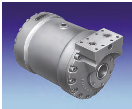
▲ Motori a pistoni assiali cilindr. fissa 1-1000 rpm 210 BAR.
