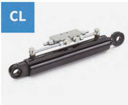
▲ Cilindri idraulici saldati - Alesaggi da 40 a 350 mm.
